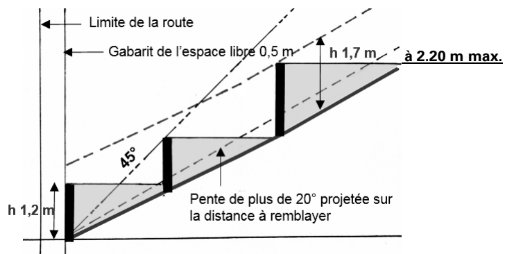
Remblayage avec terrain de référence de plus de 20°
