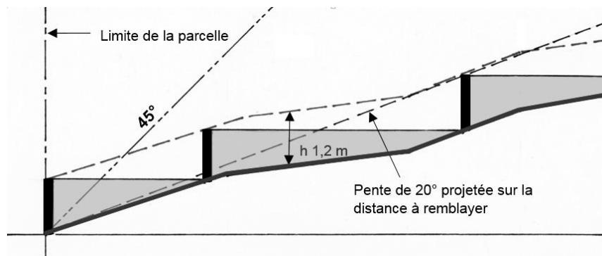
Remblayages avec mur de soutènement
